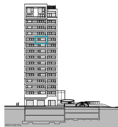
WESTGEVEL 1/1000
