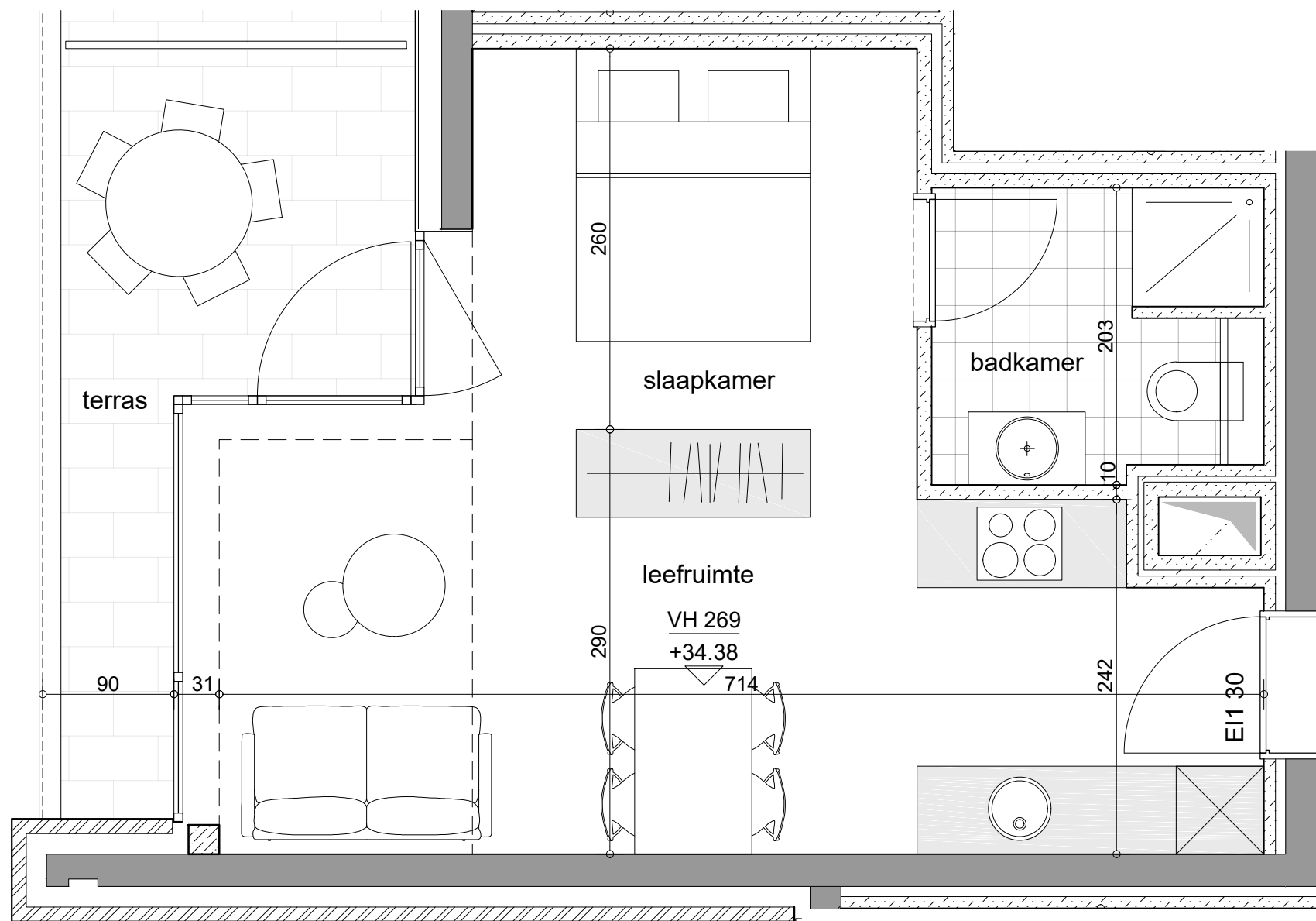
schaal 1/40
