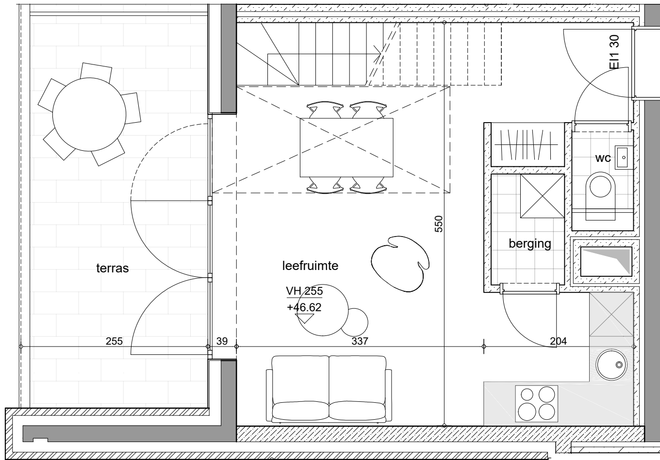
niveau +14 schaal 1/50
