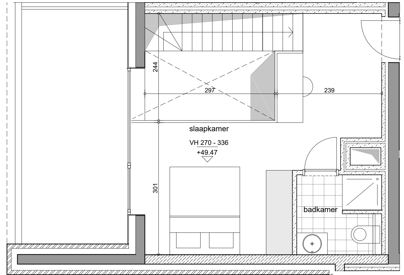
niveau +14 / duplex
