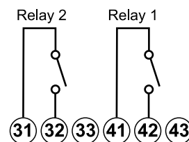
Fig. 26 Sorties à relais
